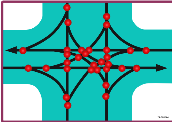
Los puntos rojos indican 32 puntos de conflicto entre vehículos en una intersección estándar de cuatro vías.
