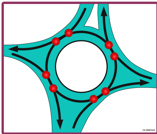
Los puntos rojos indican ocho puntos de conflicto entre vehículos en una glorieta moderna.
